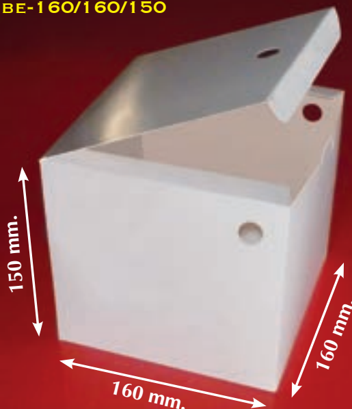
CUBE-160/160/150
